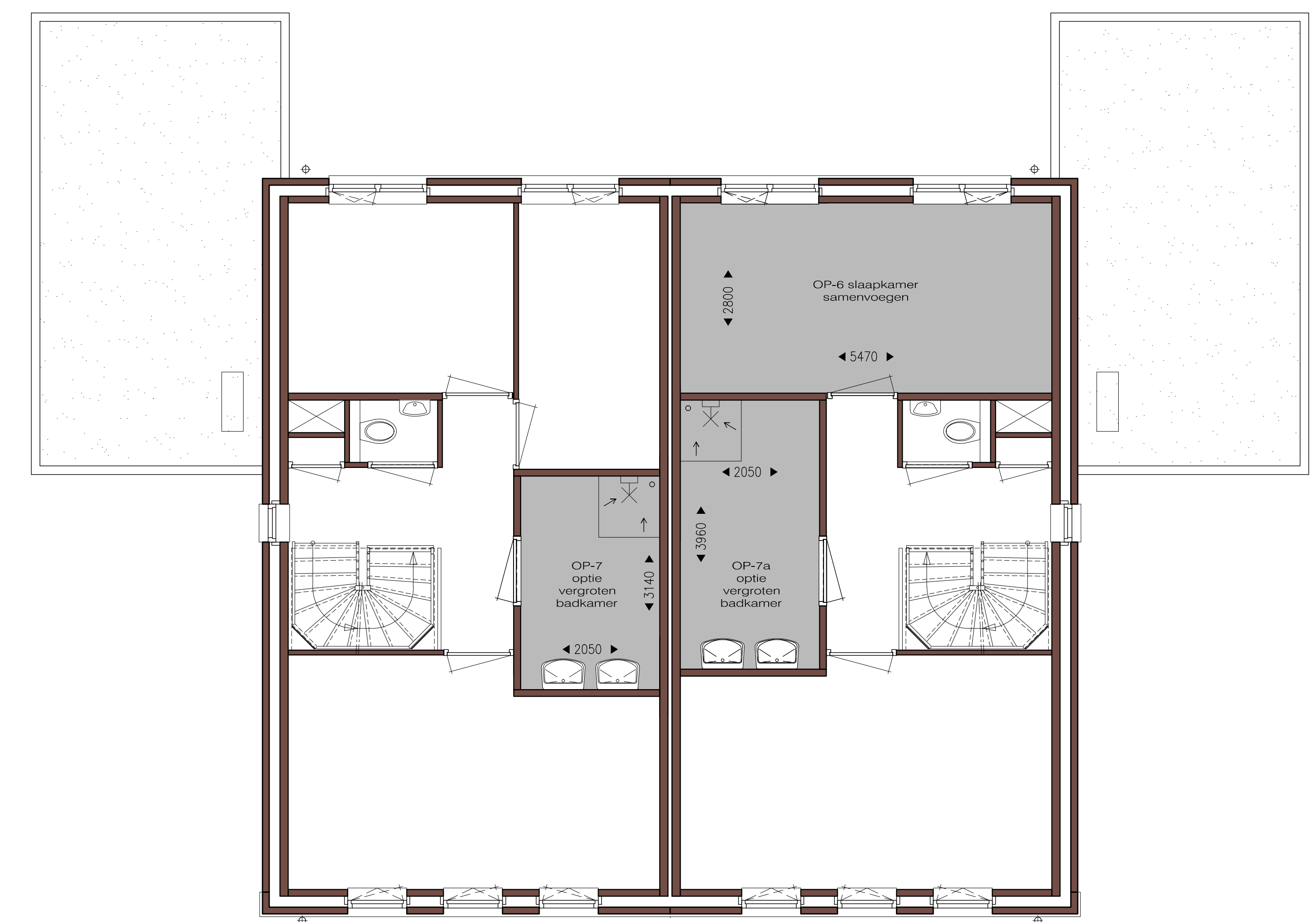
1e Verdieping
