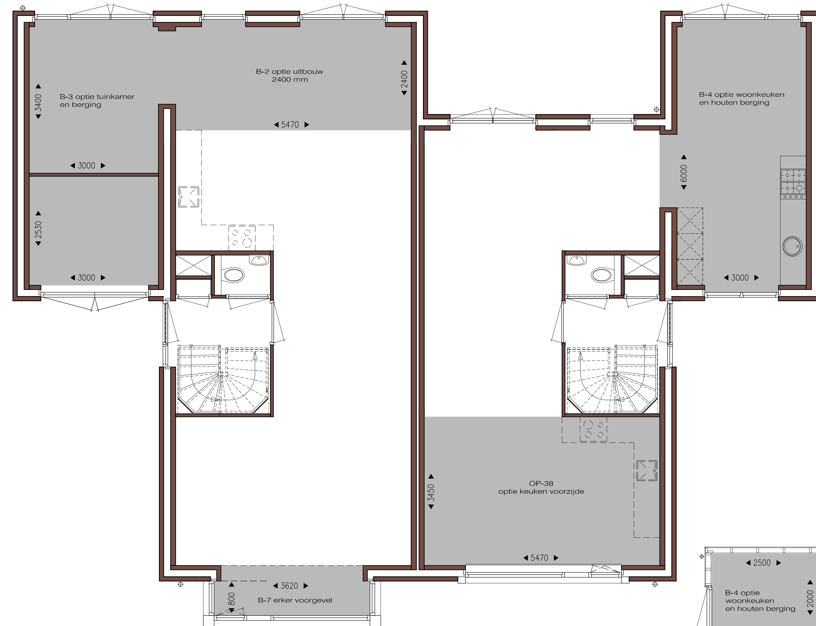
Begane grond
