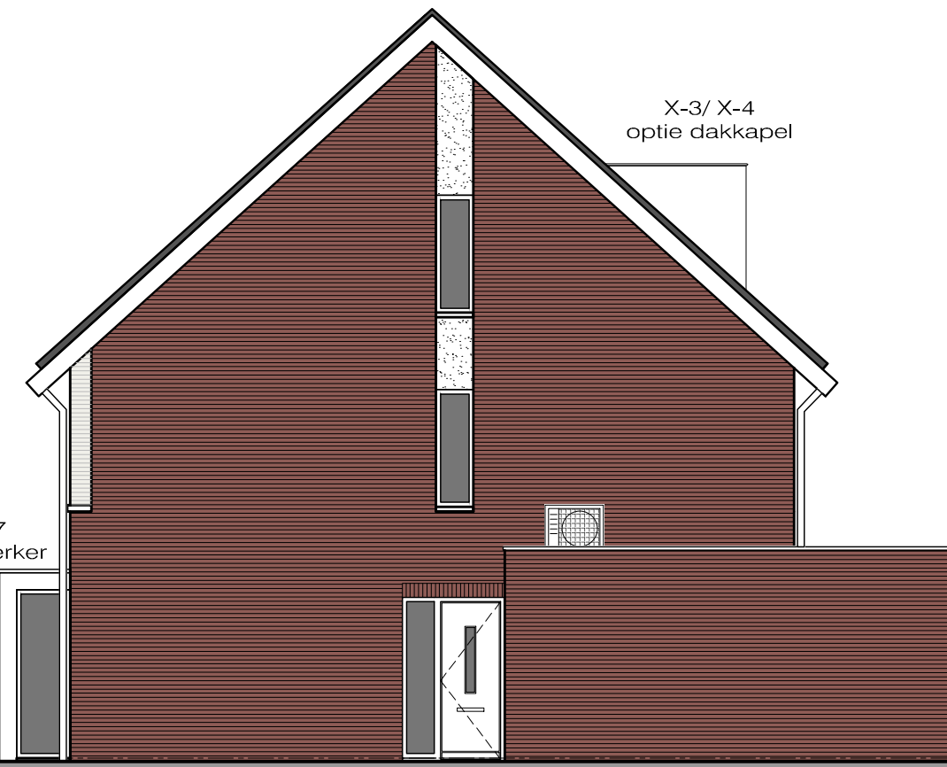
B-3/ X-4 optie dakkapel B-7 optie erker Rechter zijgevel
