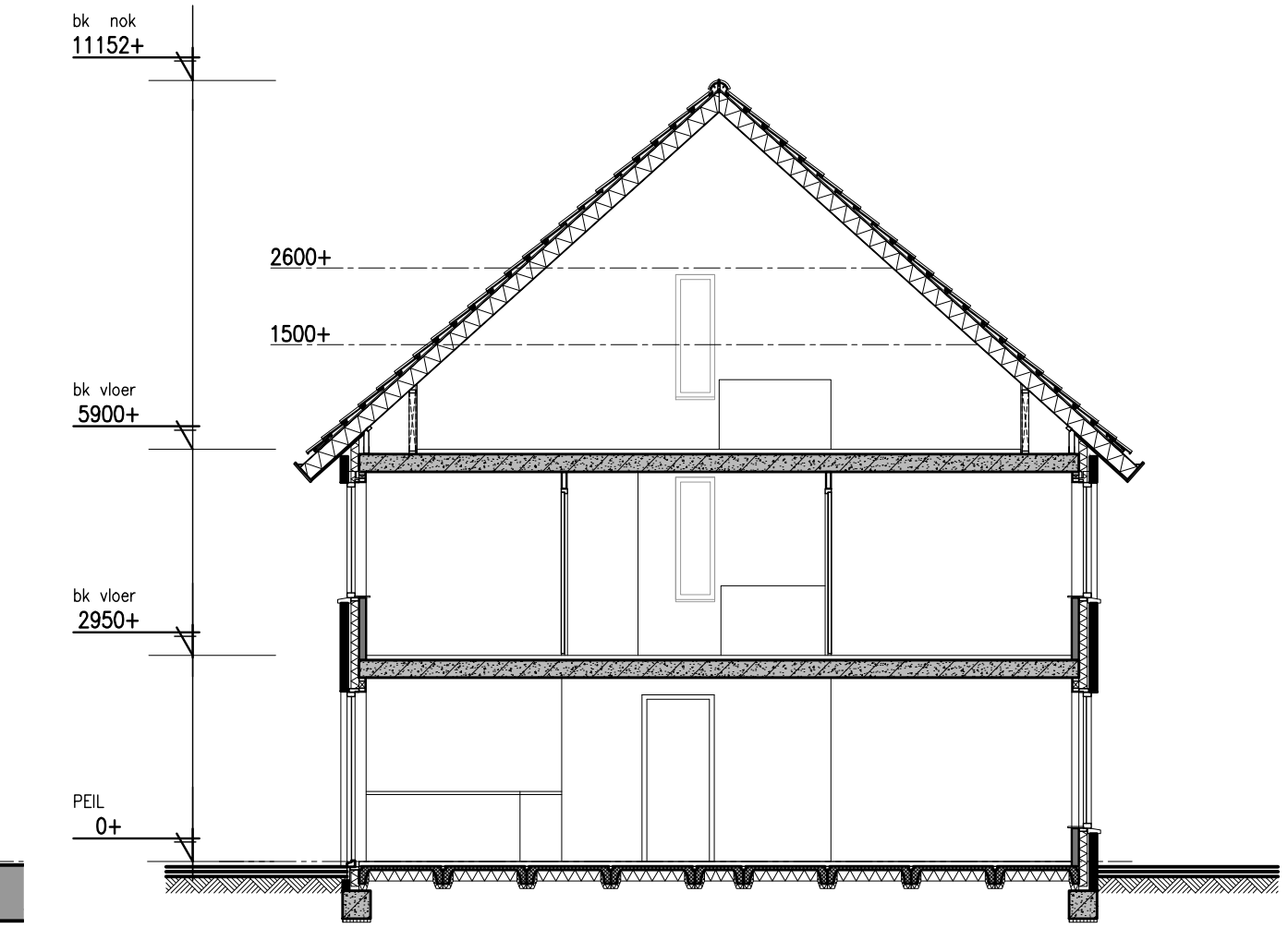
Doorsnede A-A
