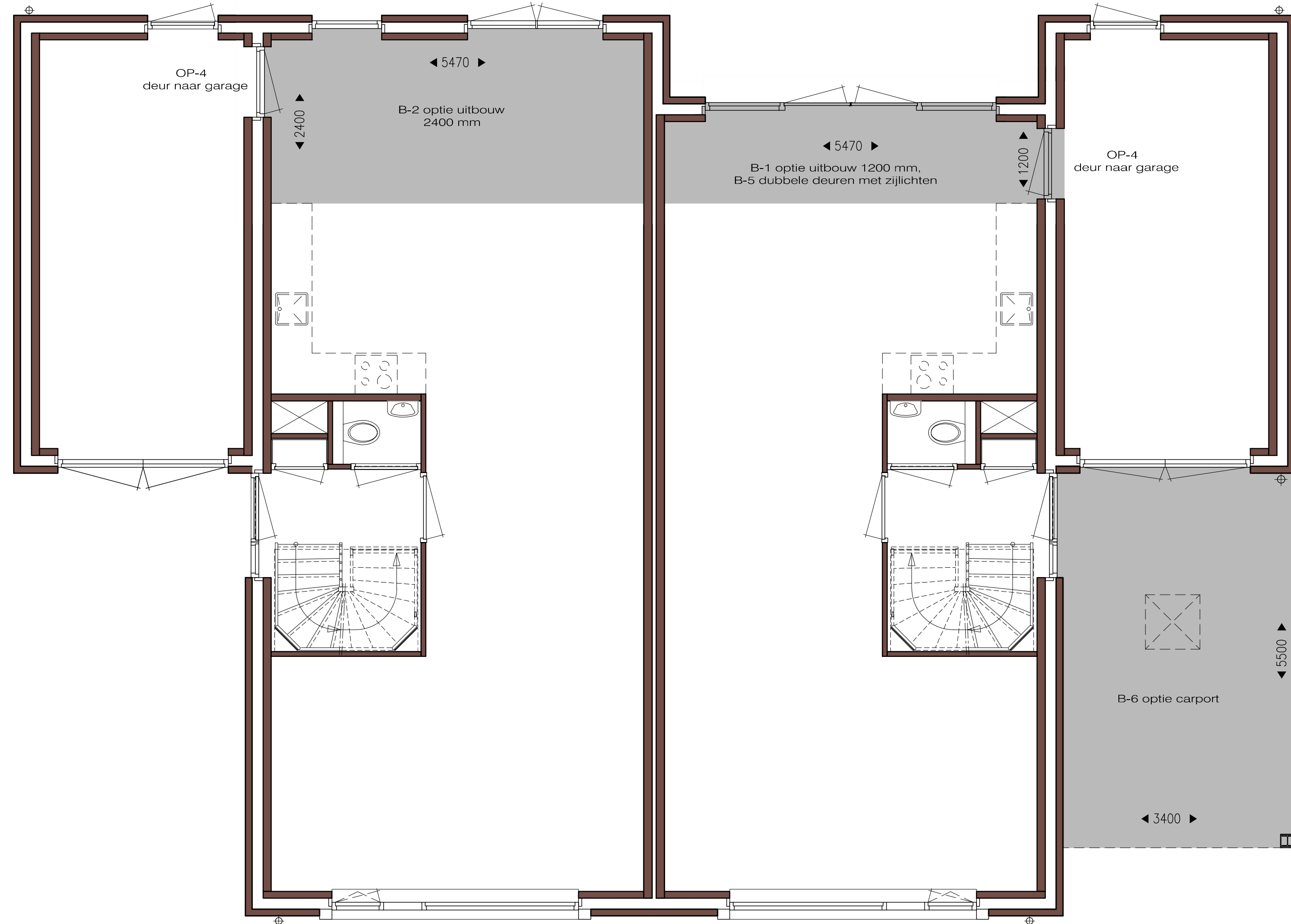
Begane grond
